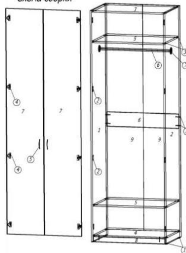
Схема сборки
