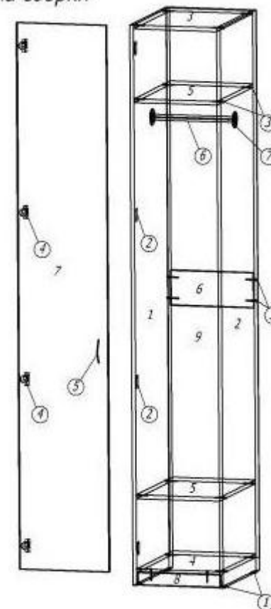
Схема сборки
